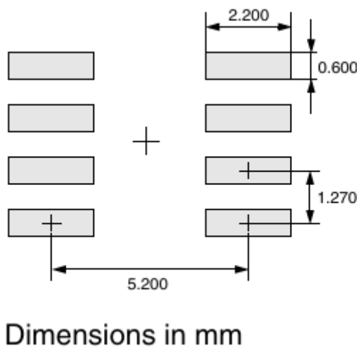
图 16 推荐的焊盘尺寸
