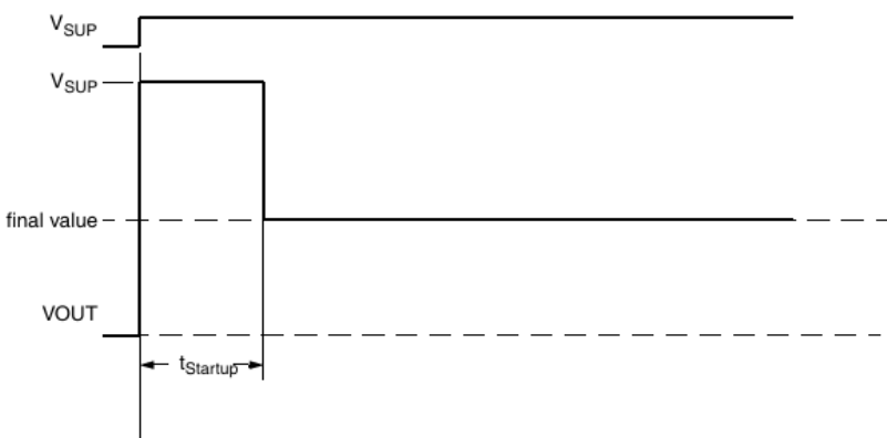
图 8 POR 定时
