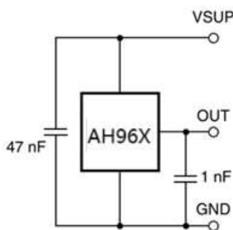
图 13 AH96X 在 PWM 模式下的推荐应用电路
